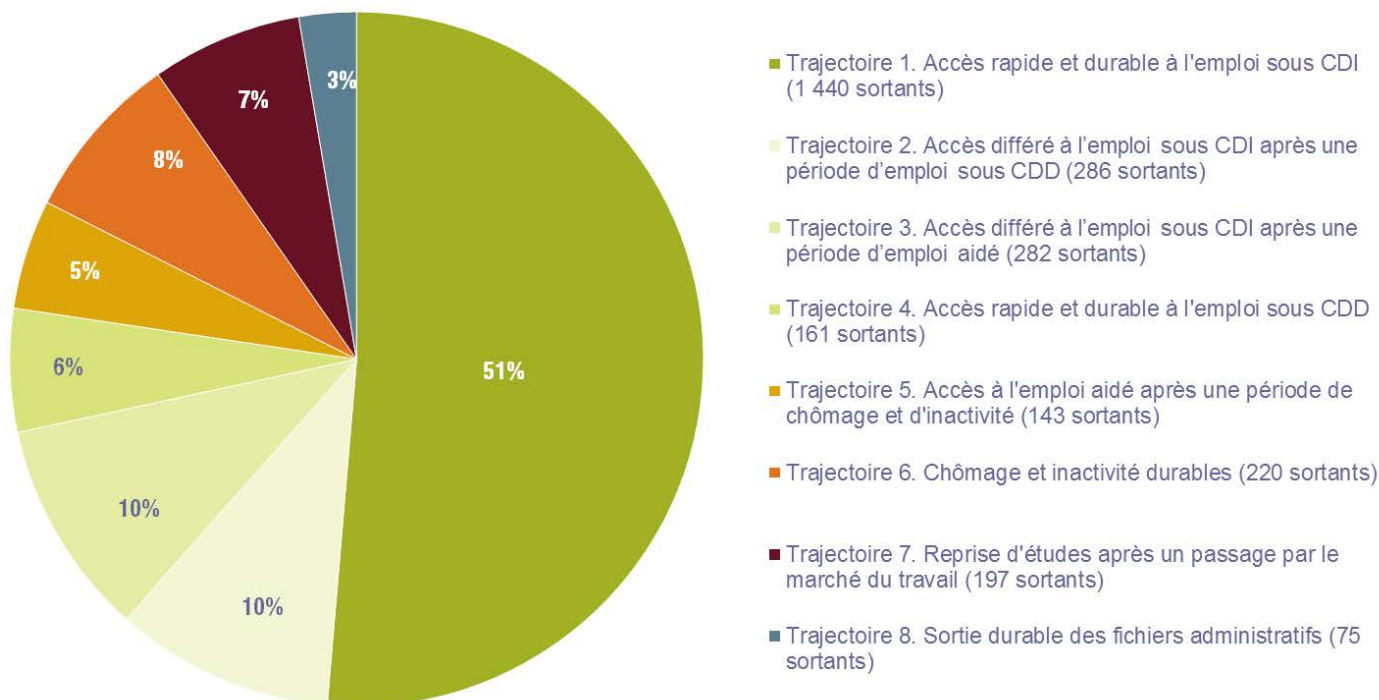
Graphique 1. Huit trajectoires types d'insertion professionnelle : répartition des sortants entre les différentes trajectoires types (en % et en nombre)
